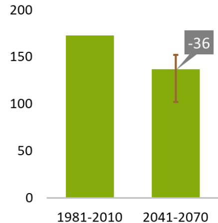
Nombre de jours avec un couvert de neige supérieur à 3 cm. La barre verticale brune représente l'incertitude. Données : Ouranos, 2017.
