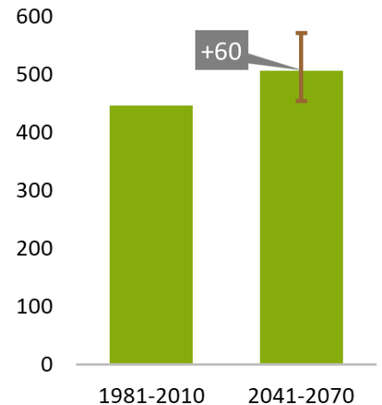
Précipitations de décembre à mai (mm).
