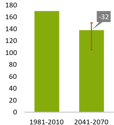
Nombre de jours avec un couvert de neige supérieur à 3 cm. La barre verticale brune représente l'incertitude. Données : Ouranos, 2017.
