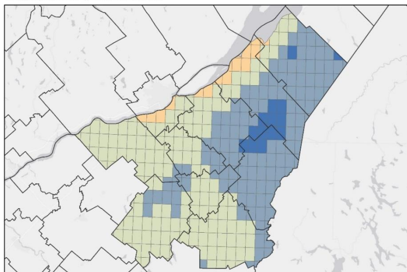
Chaudière-Appalaches - Historique 1981-2010 Températures moyennes annuelles
