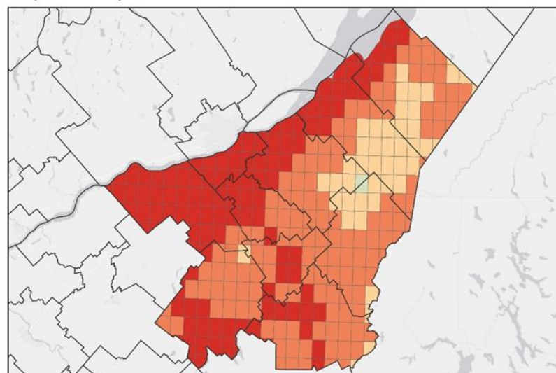
Chaudière-Appalaches - Futur 2041-2070 Températures moyennes annuelles
