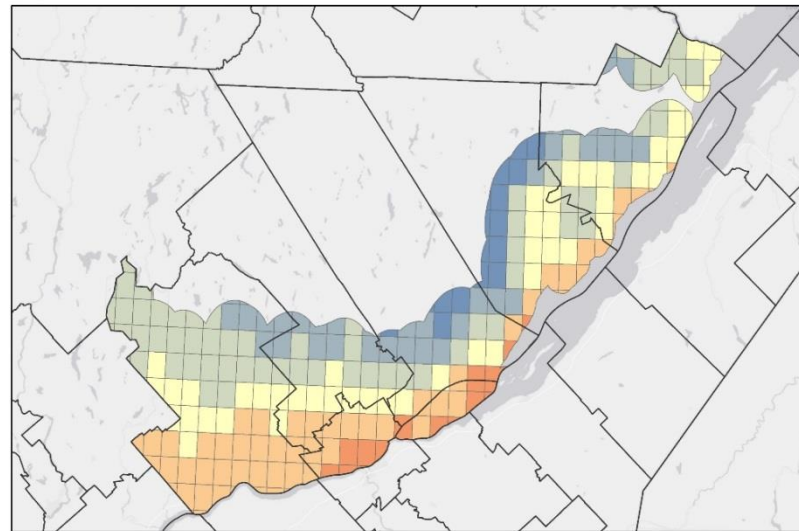
Capitale-Nationale - Historique 1981-2010 Températures moyennes annuelles
