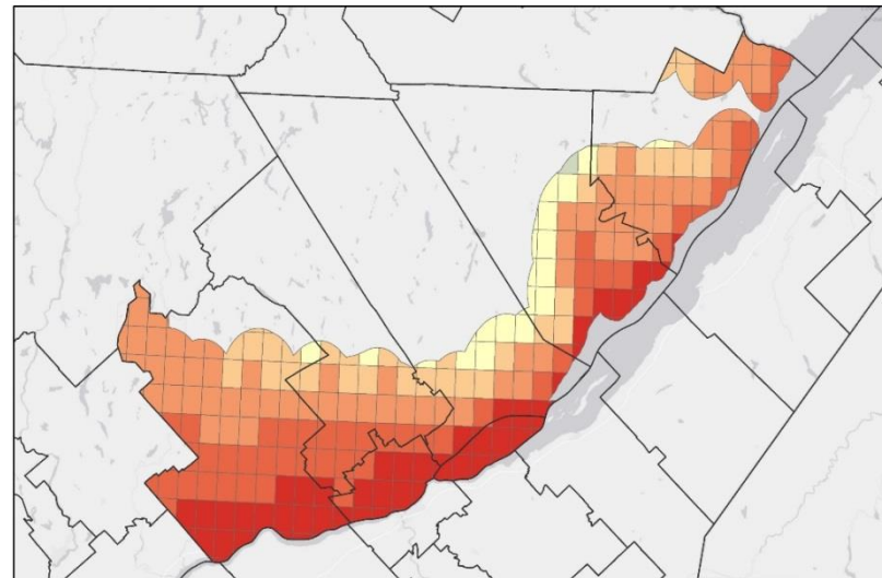
Capitale-Nationale - Futur 2041-2070 Températures moyennes annuelles
