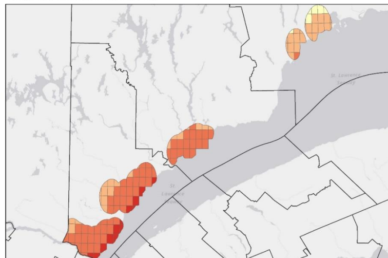
Côte-Nord - Futur 2041-2070 Températures moyennes annuelles
