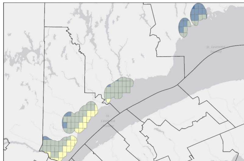
Côte-Nord - Historique 1981-2010 Températures moyennes annuelles
